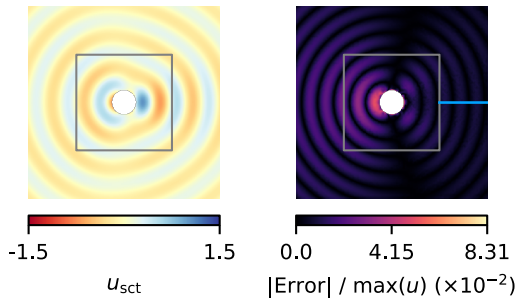
BEM - Amplitude
