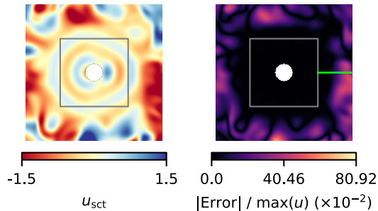
PINNs - Amplitude
