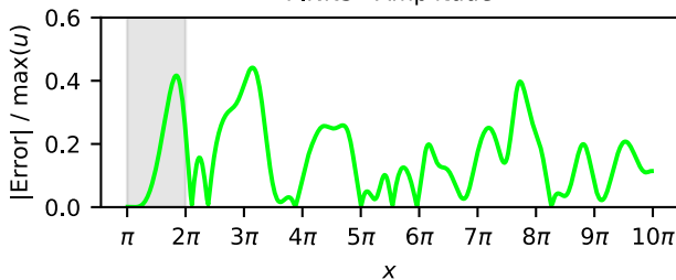
PINNs - Amplitude
