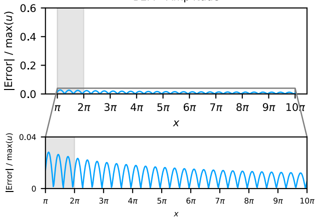
BEM - Amplitude
