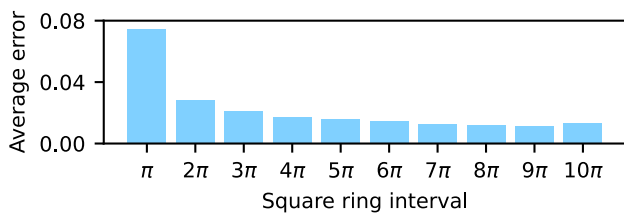
BEM - Amplitude
