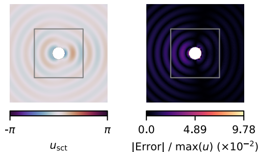
BEM - Phase
