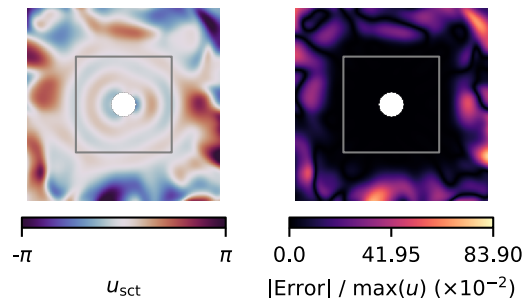
PINNs - Phase
