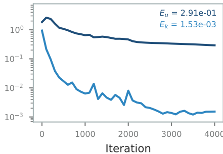
Error
