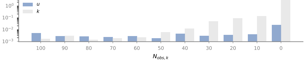
MAE
