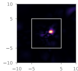
KAN
