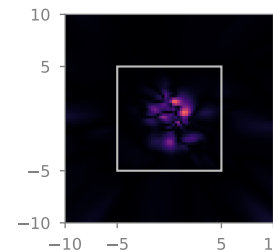
MLP
