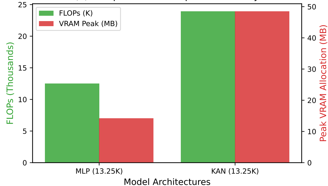
(d) Computational Footprint & Memory
