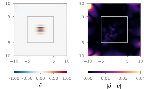
MLP
