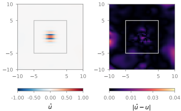
KAN
