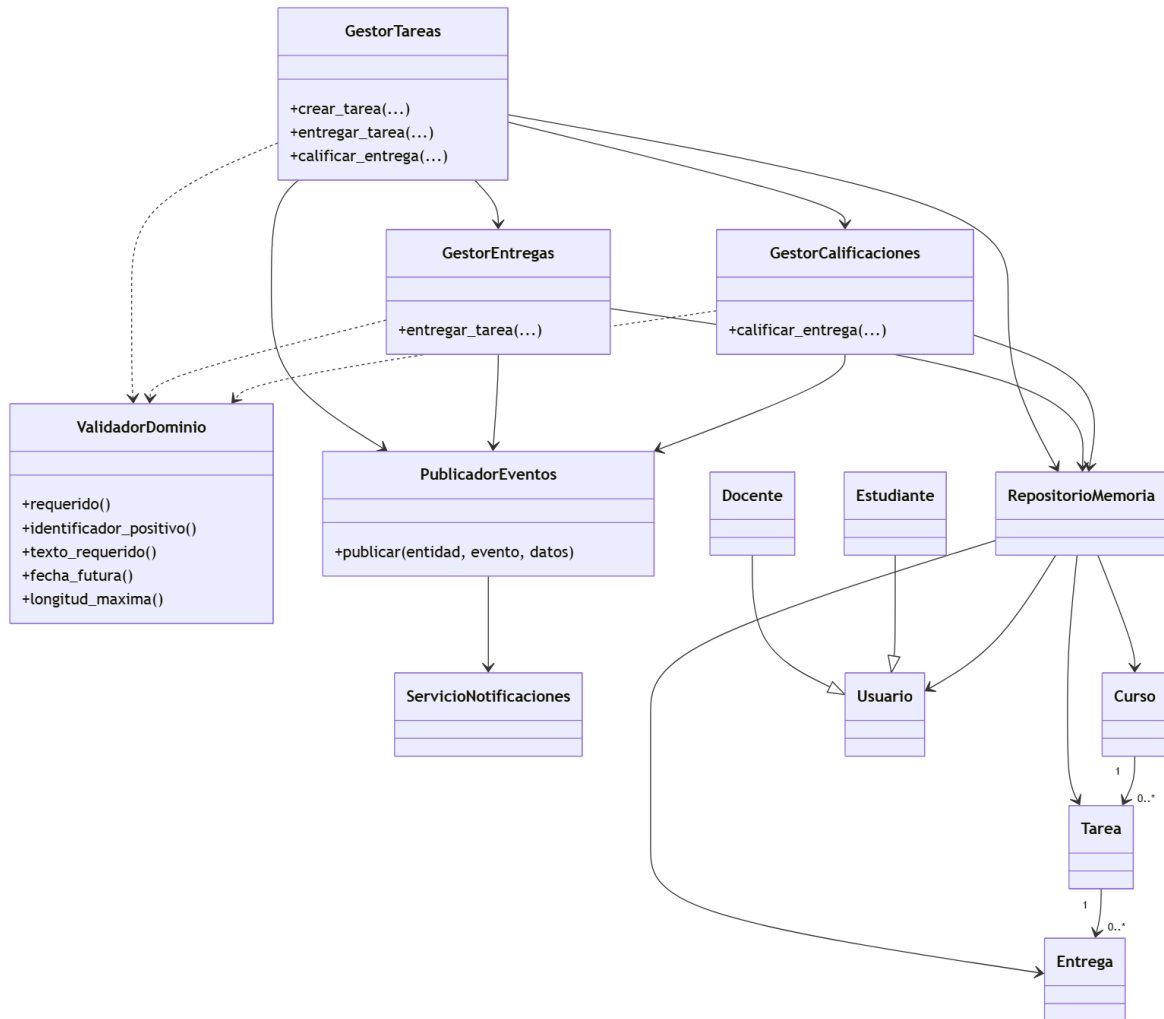
Diagrama B - Despues de las seis refactorizaciones (checkpoint fase3-refactor-domain)
