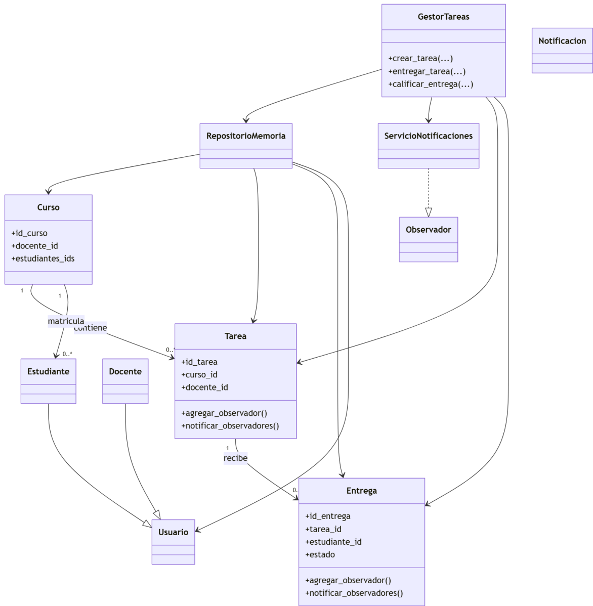
Diagrama A - Antes de refactorizar (checkpoint fase2-final)
