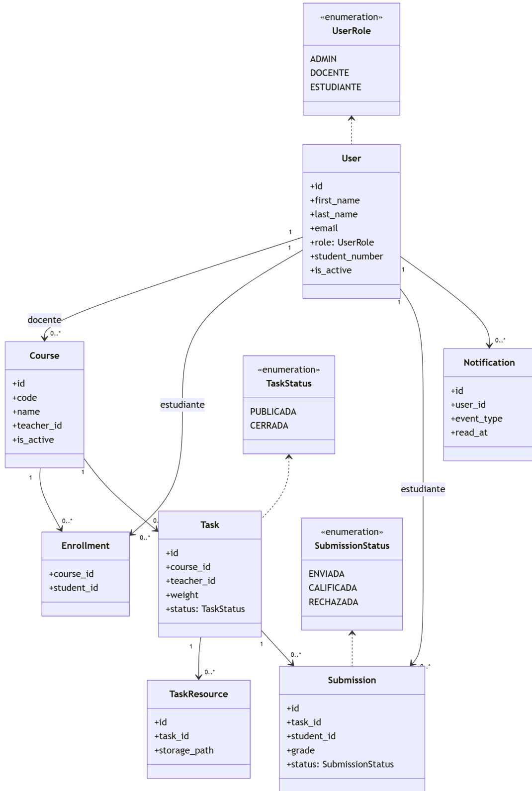
Diagrama C - Modelo final de la aplicacion web (HEAD actual)
