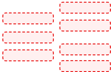
Chunks Pequeños
