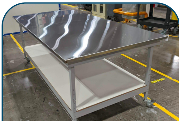
Estructura soldada, corte y doblado de acero inoxidable, corte de MDF y ensamble
