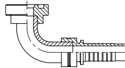
4243 Rak SAE J518 fläns Kod 61 Flänsstorlek 5/8" komatsu PRODUKTGRUPP 300
