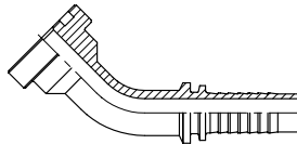
4248 45° SAE J518 fläns Kod 61 PRODUKTGRUPP 300
