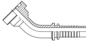
4258 45° SAE J518 fläns Kod 62
