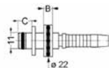
4374-11 Högtryckstvättkoppling Med lager och bricka
