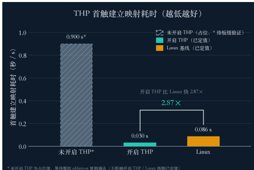
图 18: THP 提升与新建映射跳过 TLB 失效把 128 MB 私有匿名首次触碰压至 0.030 s, 快于 Linux 的 0.086 s (领先 2.87 倍)
