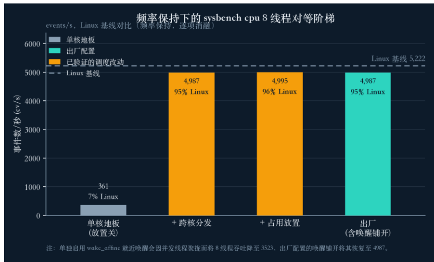
图 14: sysbench cpu 对等阶梯 (频率固定)。单核地板 (放置关闭) 约 361 ev/s, 补齐跨核分发跃至约 4987 ev/s, 占用感知放置与出厂配置在此量级持平, 分别约 4995 与 4987 ev/s, 为 Linux 5222 的 0.96 倍
