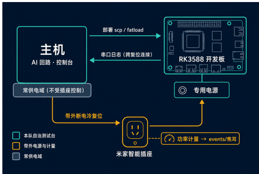
图 28: 带外电源控制的真机自治测试台：主机与串口适配器接常供电，板卡专用电源经计量式智能插座切换；暖重启为常规快路径，智能插座硬断电冷启为与被测软件状态无关的恢复原语
