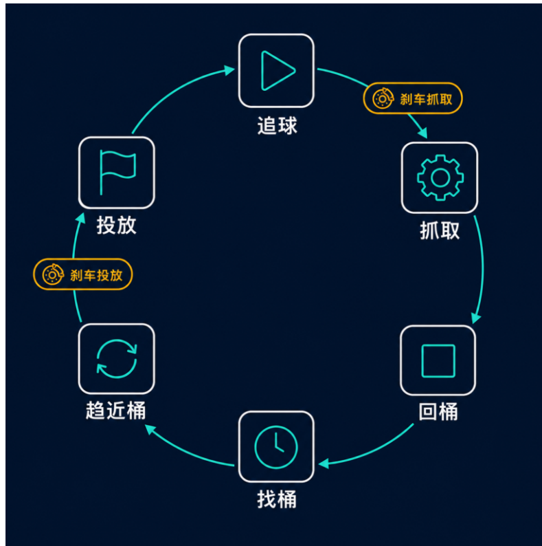
图 8: 拾球状态机：六状态非阻塞闭环，两个刹车时相由单调时钟推进，定时时相时长与相机供帧频率解耦
