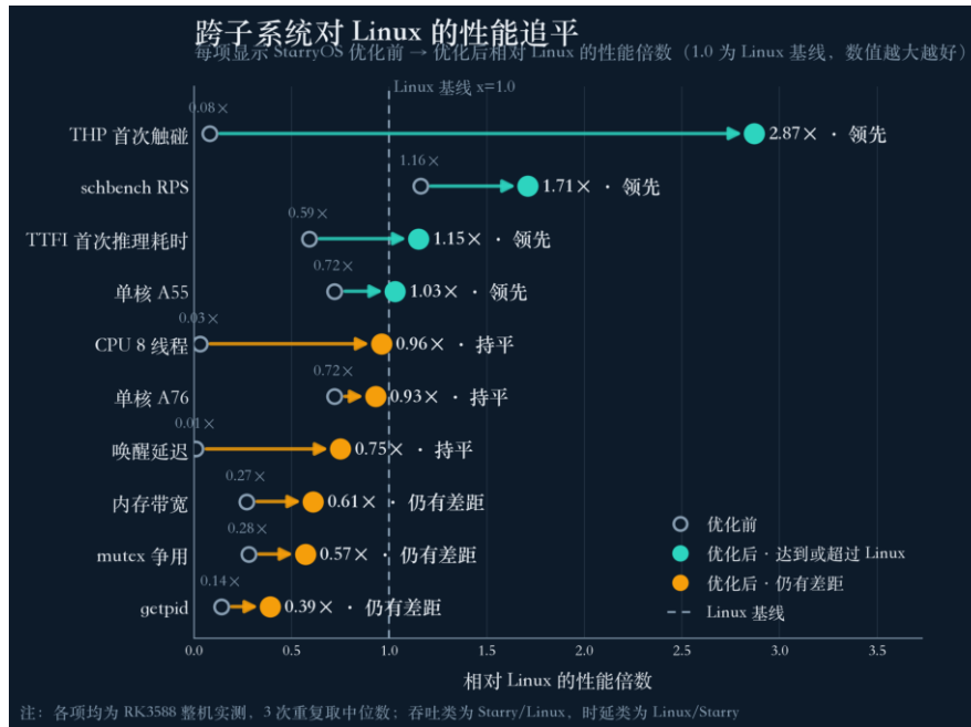
图 2：跨子系统性能追平：每项由 StarryOS 优化前（空心点）到优化后（实心点）相对 Linux 基线的性能倍数，1.0 为 Linux 基线，数值越大越好；青色为已达到或超过 Linux；橙色为尚未达到基线，分持平与仍有差距两档，见每项标注
