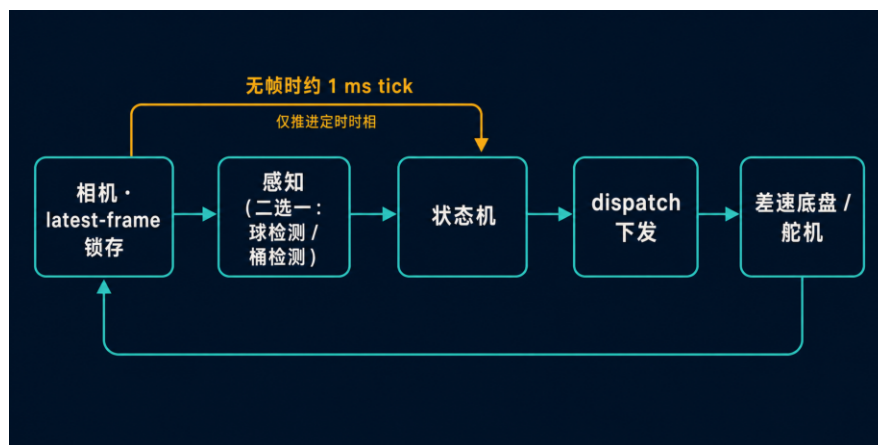
图 11: 机器人感知到控制的闭环: 相机 latest-frame 锁存、感知二选一、状态机到 dispatch 的通路, 无帧时经约 1 ms 的 tick 旁路推进定时时相
