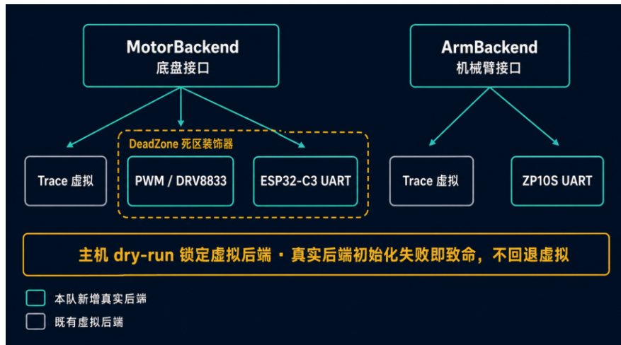
图 9：执行器分层：MotorBackend 与 ArmBackend 接口下挂 Trace、PWM/DRV8833、ESP32-C3 UART 与 ZP10S UART 四个后端，主机 dry-run 锁定虚拟路径，真实后端初始化失败即致命
