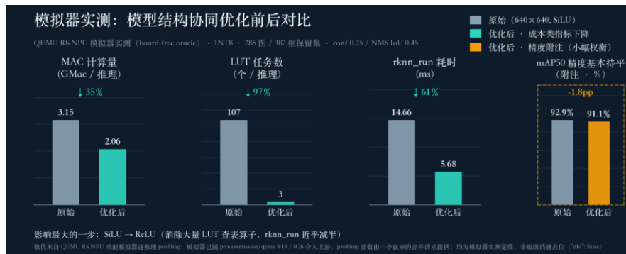
图 26: 模拟器实测: 网球模型结构协同优化把 MAC 3.15→2.06 GMac、LUT 任务 107→3、rknn_run 14.66→5.68 ms, 同时 mAP50 保持在 92.9→91.1%
