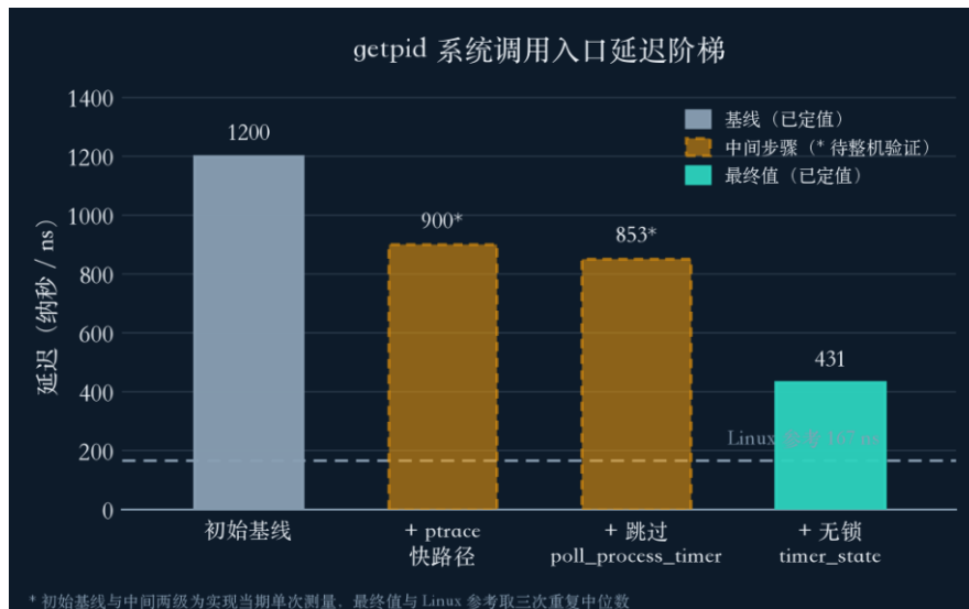
图 16: getpid 三步累计从 1200 ns 降到 431 ns，为 Linux 167 ns 的 2.6 倍，残余逼近 uctx.run 的陷入下限
