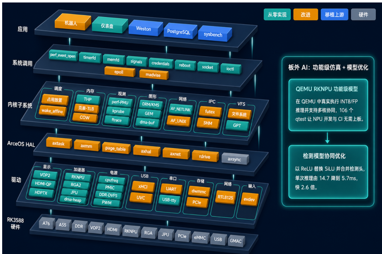
图 4：内核贡献全景：自机器人应用向下至 RK3588 硬件，本队在每一层的贡献按角色着色，绿为从零实现、橙为改进、蓝为移植使能上游软件、灰为复用硬件；右侧另列板外 QEMU RKNPU 功能级模型与检测模型的协同优化。
