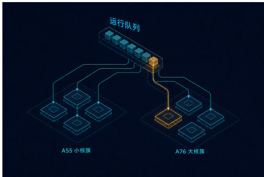
图 13: axtask 放置管线，青色为新增实现；顶部为待放置线程，各核持私有运行队列。派生分发在亲和性允许的核间轮转，单原子 occ 占用计数供派生与唤醒共用并每 tick 自愈，wake_affine 在唤醒者空闲时把被唤醒者就近交回，共同把负载在大小核间铺开
