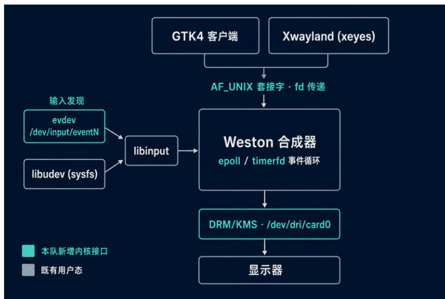
图 24: Weston 于 StarryOS: 客户端经 AF_UNIX 套接字连入并提交窗口缓冲，输入沿 libinput 与 libudev 自 sysfs 与 evdev 发现，DRM/KMS 承载扫描输出，整套事件经 epoll 与 timerfd 汇聚轮转
