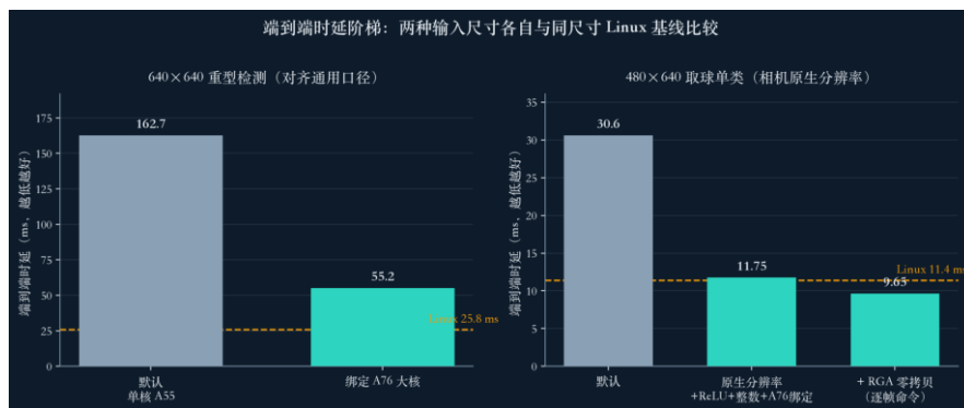
图 6: 两种输入尺寸各自的端到端时延阶梯，各与对应尺寸的 Linux 基线比较
