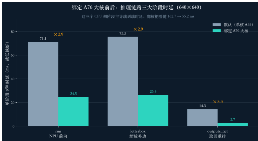
图 7：绑定 A76 大核前后推理链路三大阶段的 p50 时延 (640×640)：run、letterbox、outputs_get 三个 CPU 侧阶段主导端到端时延，绑核将整链端到端时延由 162.7 ms 降至 55.2 ms，三段各降约 2.9、2.9、5.3 倍
