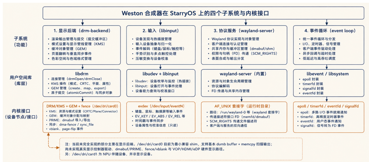
图 15 Weston 14 在 Starry 上以 DRM 加 pixman 软件后端启动, 客户端经 AF_UNIX 套接字连入并提交窗口缓冲, 输入沿 libinput 与 libudev 自 sysfs 与 evdev 发现, 整套事件经 epoll 与 timerfd 汇聚轮转
