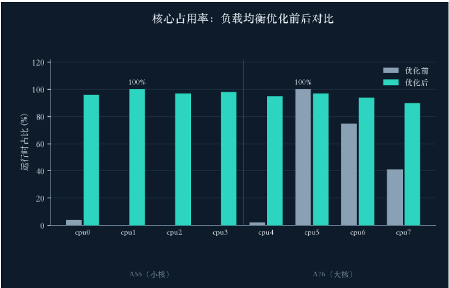
图 14: 核驻留直方图。放置均衡前八个线程集中在三个 A76 核、A55 集群近乎空闲, 唤醒接入占用信号后在 A55 与 A76 八核间均匀铺开
