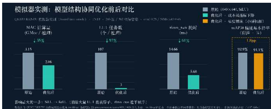
图 25: 模拟器实测: 网球模型结构协同优化把 MAC 3.15→2.06 GMac、LUT 任务 107→3、rknn_run 14.66→5.68 ms, 同时 mAP50 保持在 92.9→91.1%
