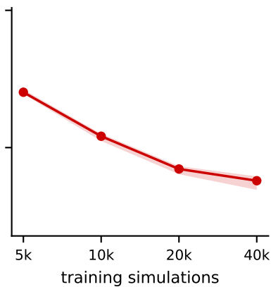
Ornstein-Uhlenbeck (vs MCMC)
