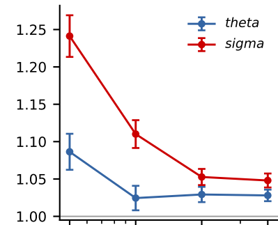
Ornstein-Uhlenbeck (vs MCMC)
