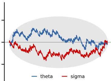
Ornstein-Uhlenbeck
