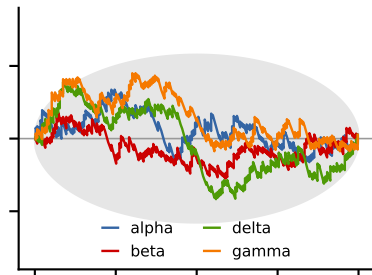
SINDy-SDE
