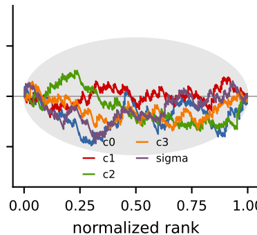
SINDy-SDE
