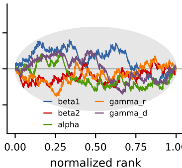
SEIR
