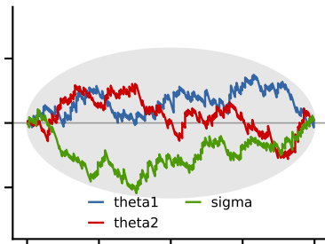
SEIR
