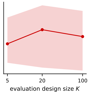
Merton jump-diffusion
