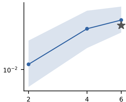
Merton jump-diffusion
