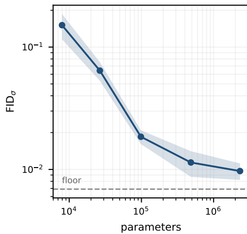
SEIR
