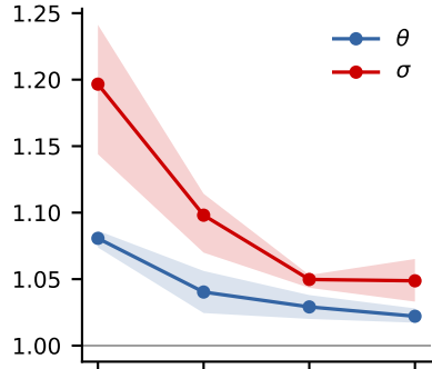
Ornstein-Uhlenbeck (vs MCMC)
