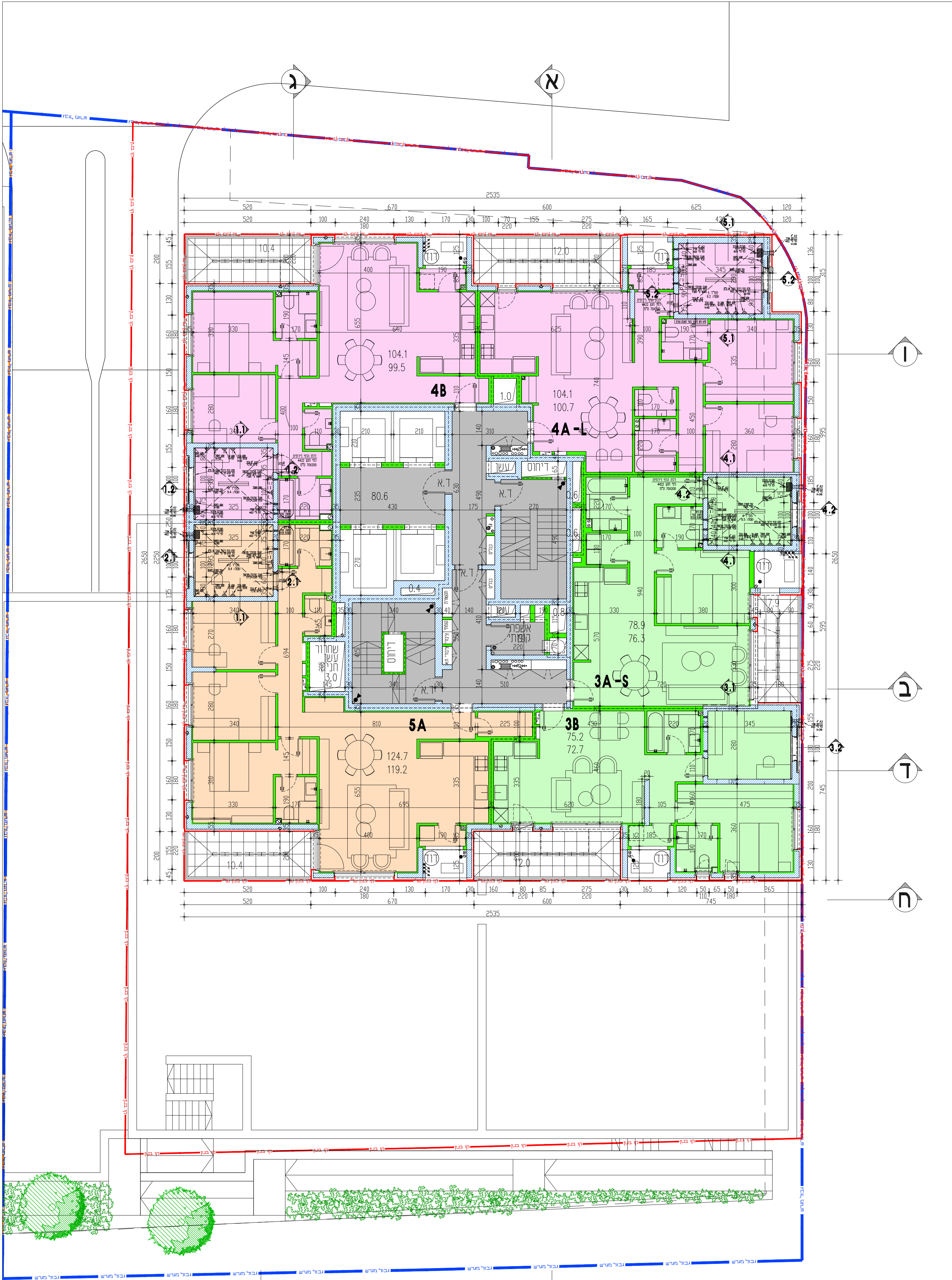
תכנית קומה טיפוסית א' קומות 2, 4, 6, 8, 10, 14, 16, 18, 20, 22
