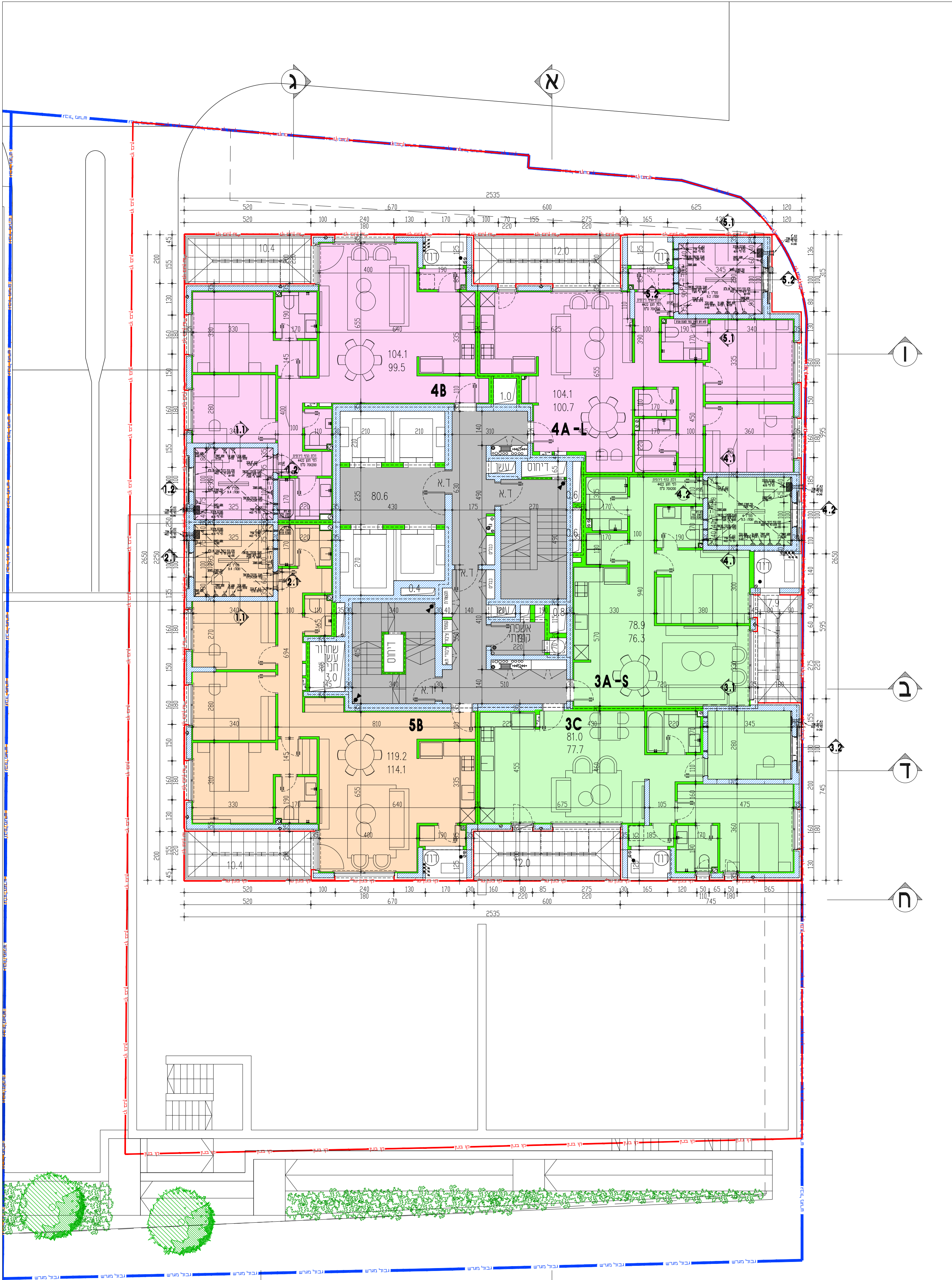
תכנית קומה טיפוסית ב' קומות 3, 5, 7, 9, 13, 15, 17, 19, 21
