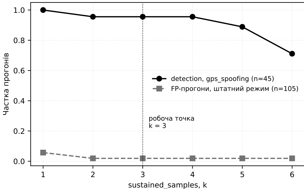
Чутливість до правила стійкості детектора
