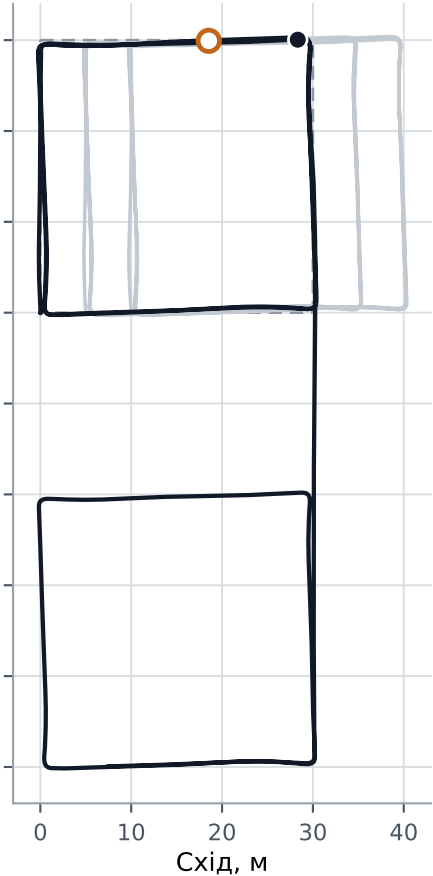
В — сегментована
