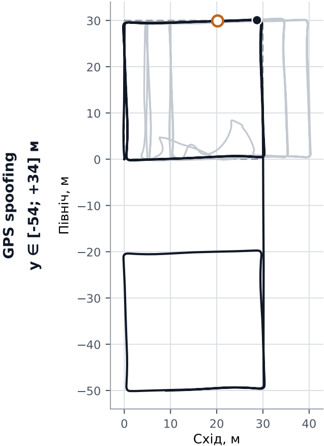
А — централізована
