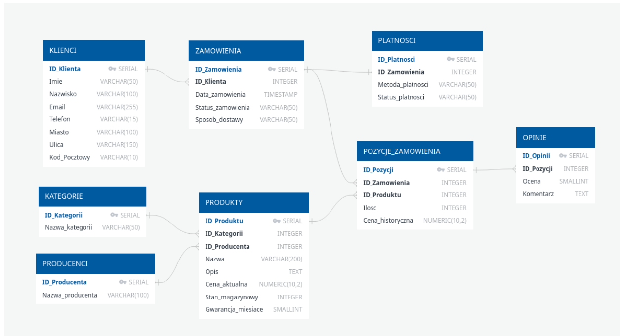
Figure4: Rysunek 4: Fizyczny schemat bazy danych opracowany dla silnika PostgreSQL.
