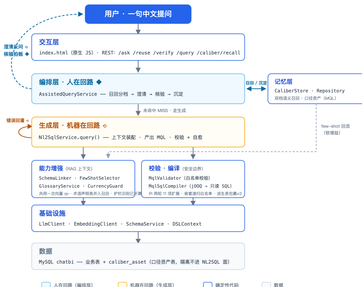
图 24 引擎层逻辑架构：主干自上而下为一次查询穿过的层；编排层（蓝）外挂记忆层，「召回 / 沉淀」双向；few-shot 回流虚线是沉淀的软增益通道；左侧两个回环即人在回路（澄清 / 核验）与机器在回路（错误回灌）
