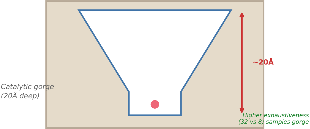
AChE (PDB 4EY7)
