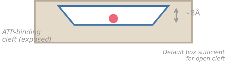
EGFR (PDB 1M17)
