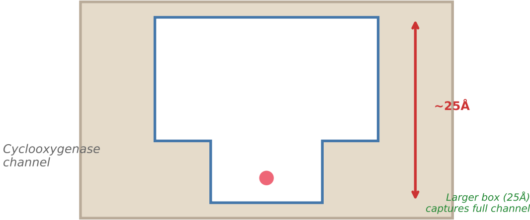
COX-2 (PDB 3LN1)
