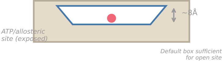
p38 (PDB 1KV2)
