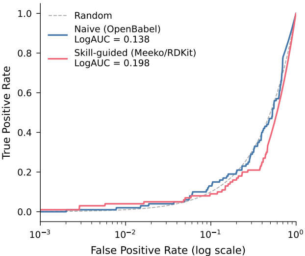
Semi-log ROC -- ache
