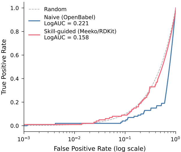
Semi-log ROC -- bace1
