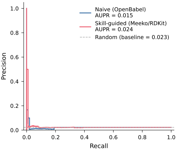
Precision-Recall -- bace1
