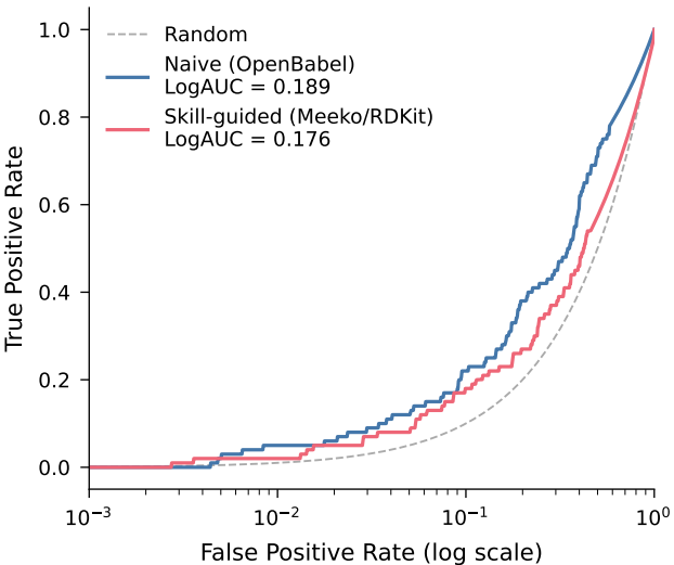
Semi-log ROC -- cdk2
