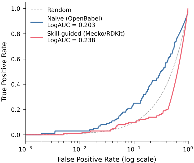
Semi-log ROC -- cox2
