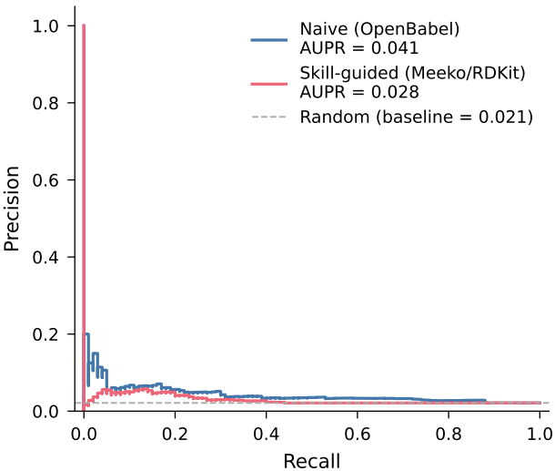
Precision-Recall -- egfr
