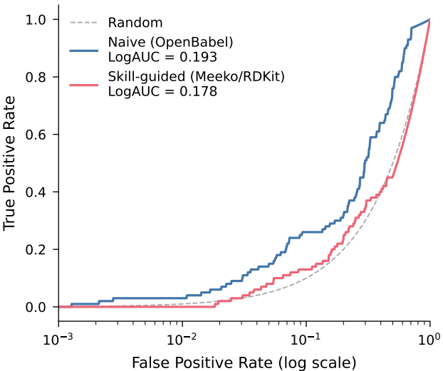
Semi-log ROC -- esr1
