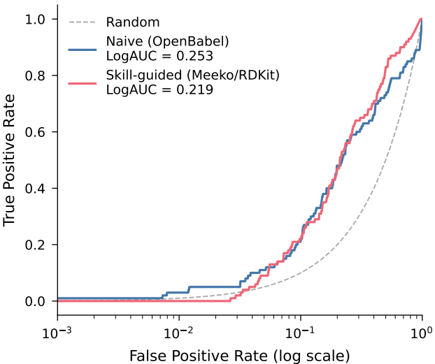
Semi-log ROC -- FPR2
