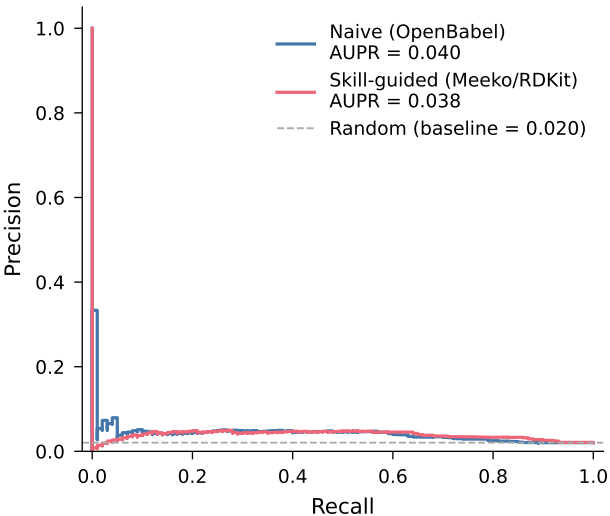
Precision-Recall -- FPR2
