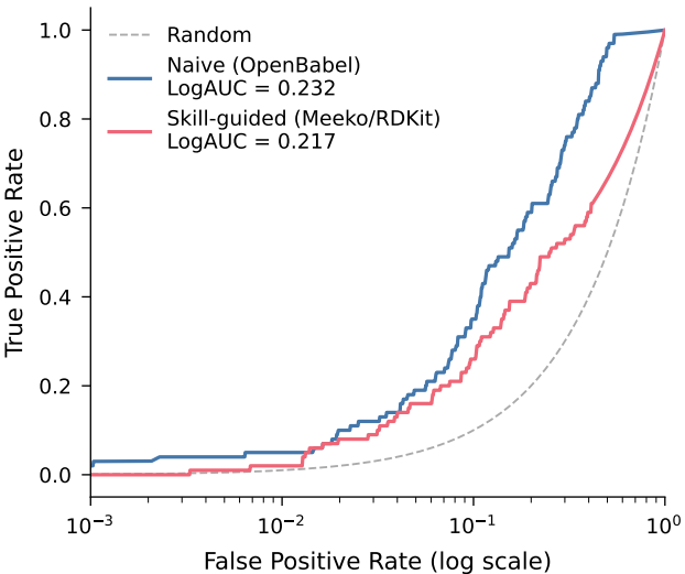
Semi-log ROC -- p38
