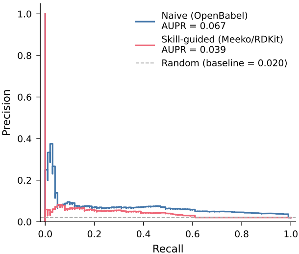
Precision-Recall -- p38
