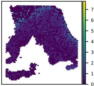
SNU18A NT5E expression Moran's I = 0.24
