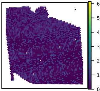
SNU27A PIDD1 expression Moran's I = 0.04
