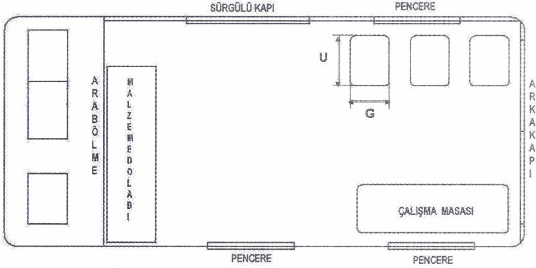
Şekil-1: Araç yerleşim planı.
