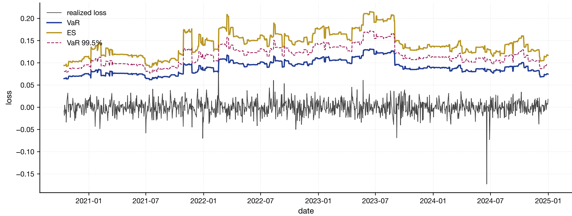
VaR / ES path — Mkt-RF
