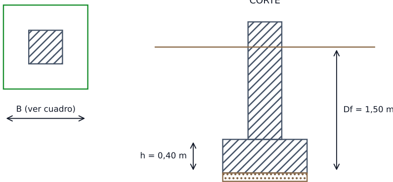
B. Zapata Z-1 (marquesina)
