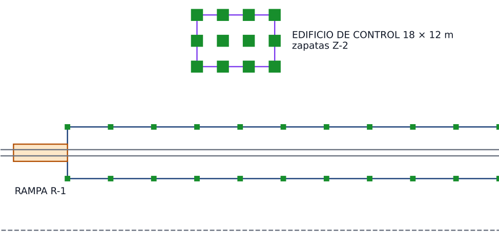
A'. Detalle del extremo de la terminal (rampa, primeros pórticos y edificio)
