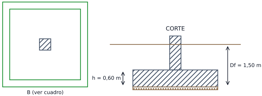
C. Zapata Z-2 (edificio de control)
