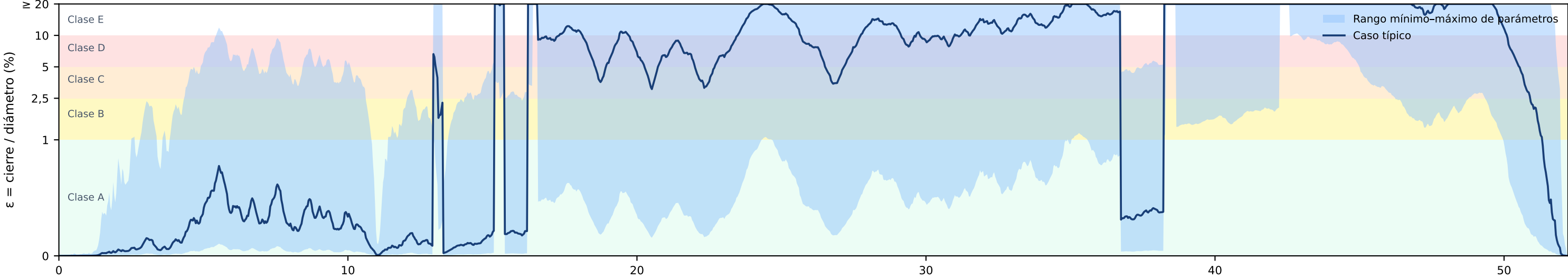
C. Aptitud para tuneladora de doble escudo (verde favorable · ocre condicionada · rojo desfavorable → método convencional)
