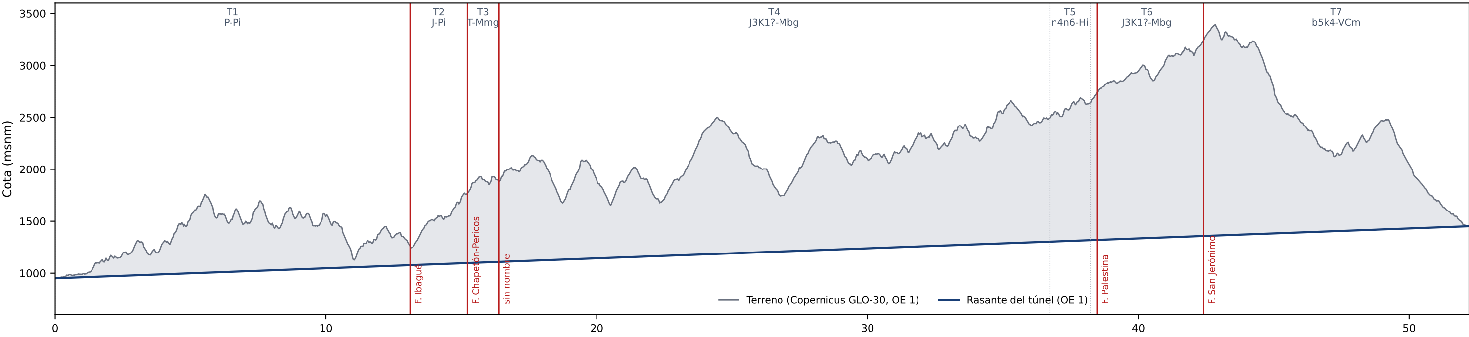
A. Perfil longitudinal con tramos litológicos (MGC 2023) y fallas cartografiadas — PK en km desde el portal oriental (Ibagué)
