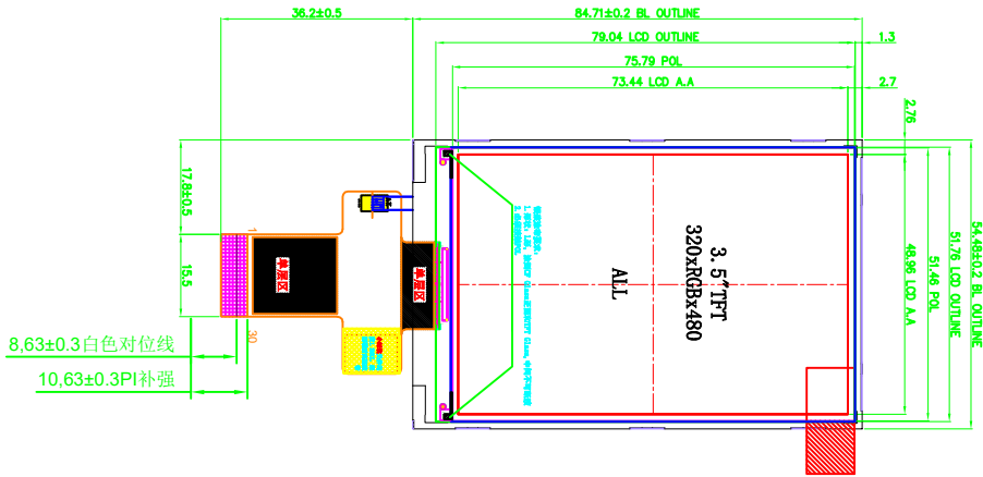
正视图
