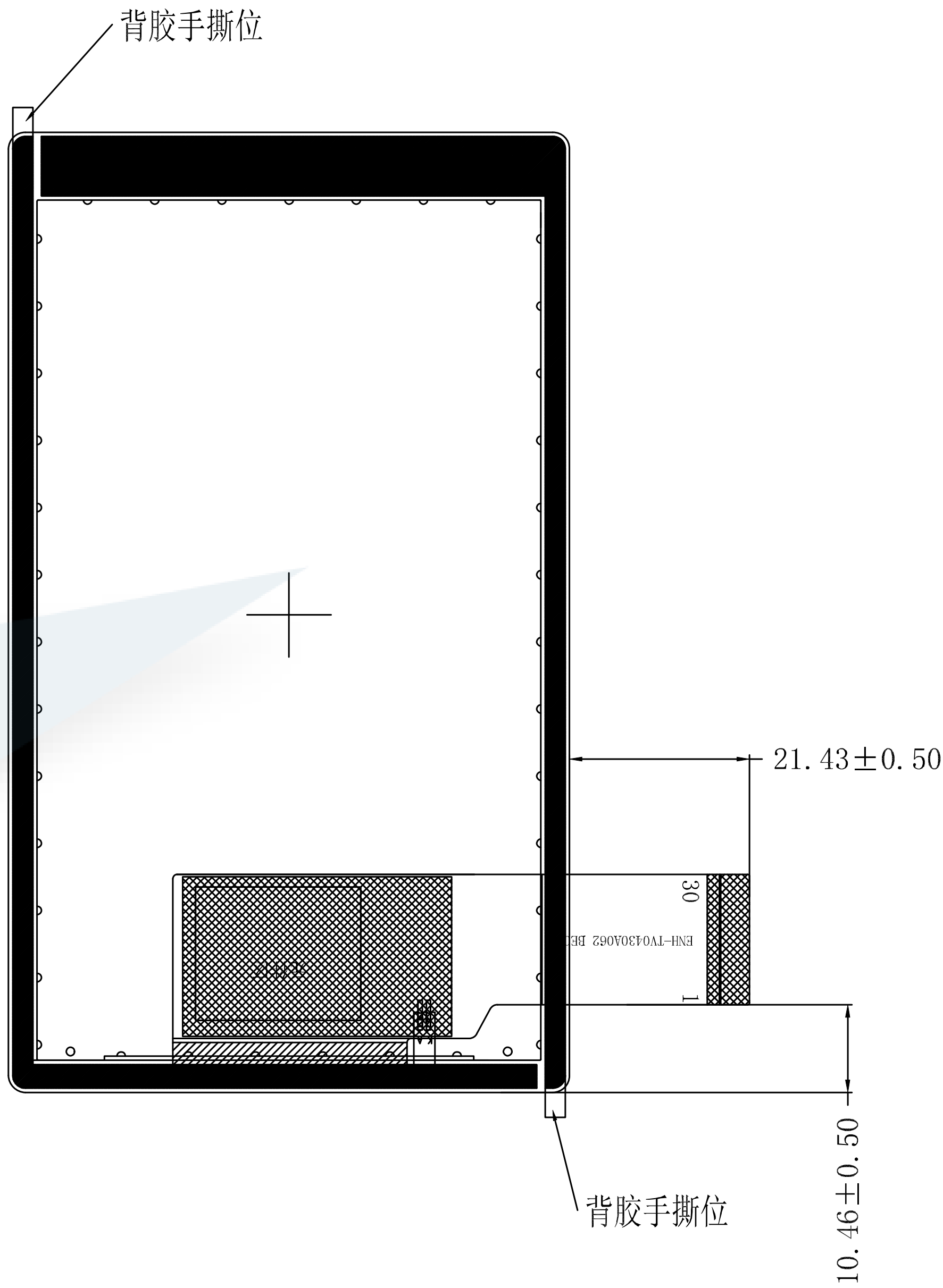
FPC弯折示意图 总成FPC弯折粘贴出货
