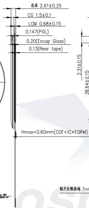
侧视图
