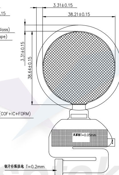
背视图
