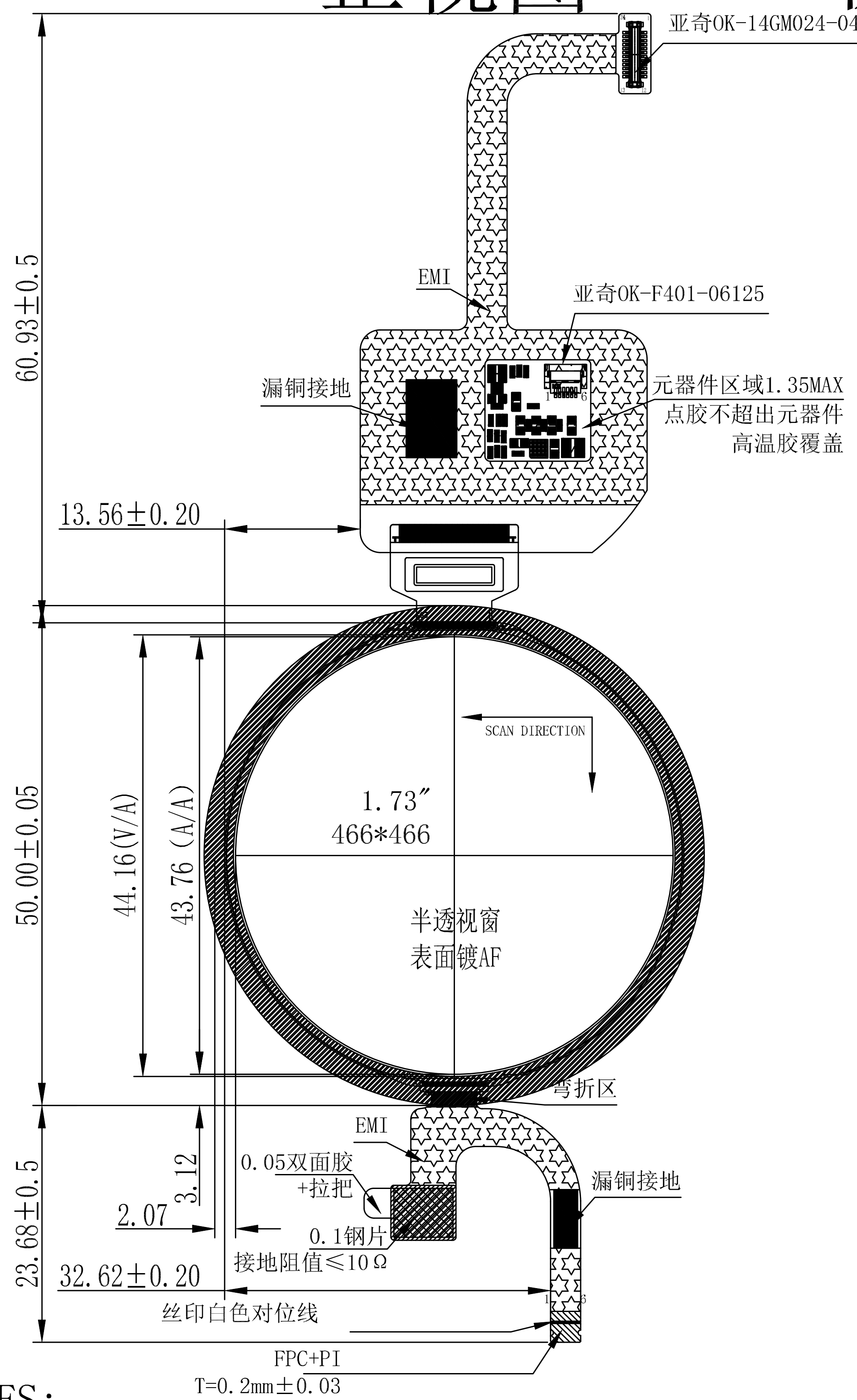
正视图
