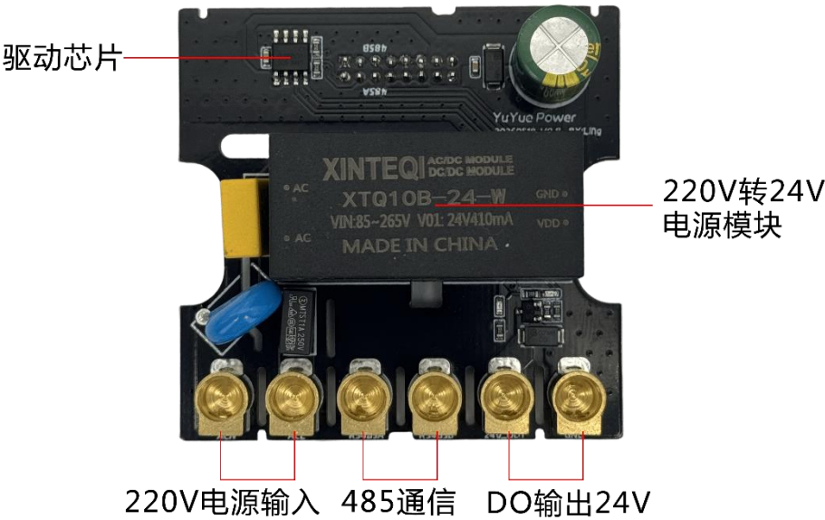
背面 220V 电源模块及接口
