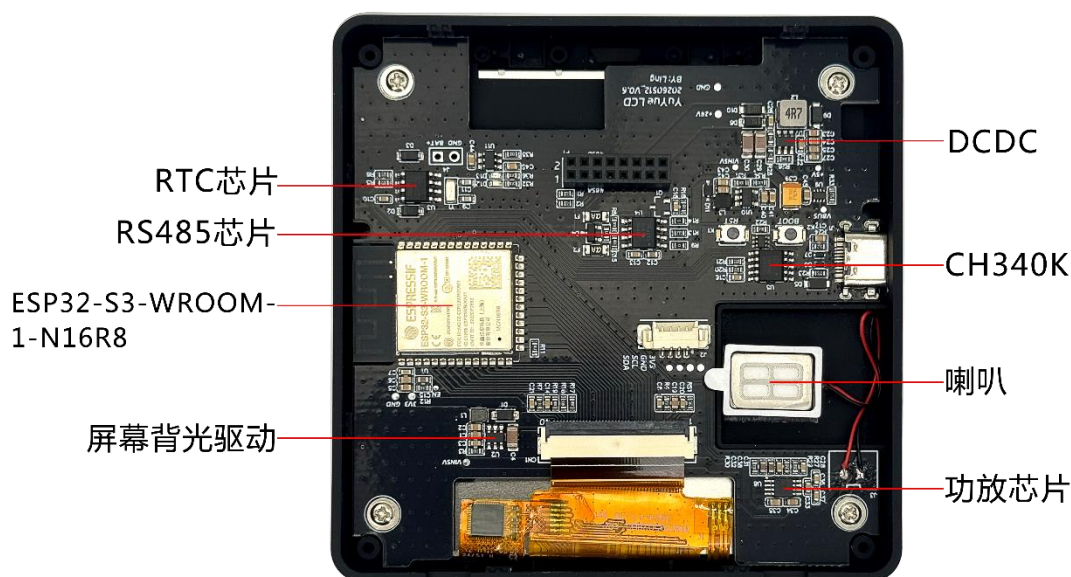
正面结构及主要功能标注
